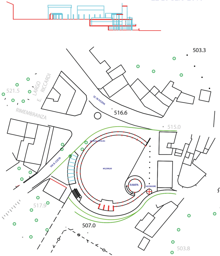
LIVELLO PIAZZA DELLA LIBERTA' 0,00 scala 1:500
