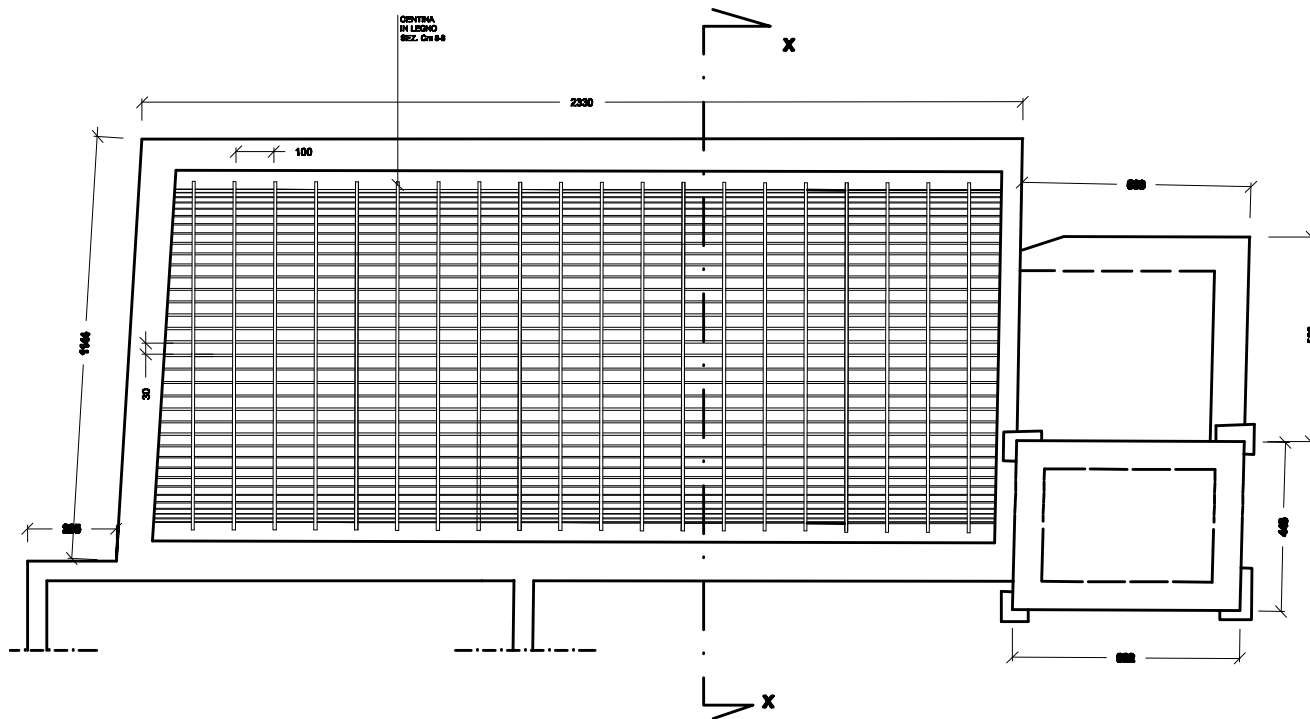
PIANTA DELLA CENTINATURA DELLA VOLTA IN CANNE E GESSO
