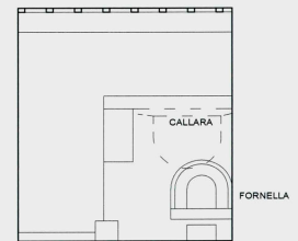
SEZIONE TRASVERSALE PROSPETTO DELLA CALLARA
