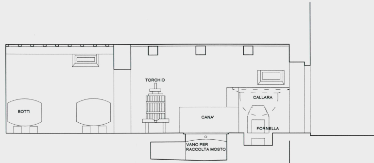
SEZIONE LONGITUDINALE
